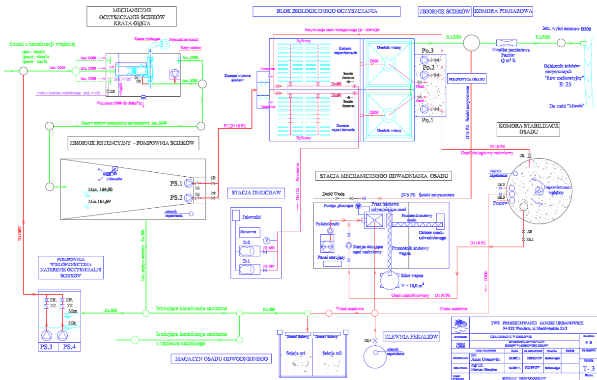
SCHEMAT TECHNOLOGICZNY - PRZEBUDOWA O.Ś W MIEJSCOWOŚCI CEGŁÓW (4500 RLM)
